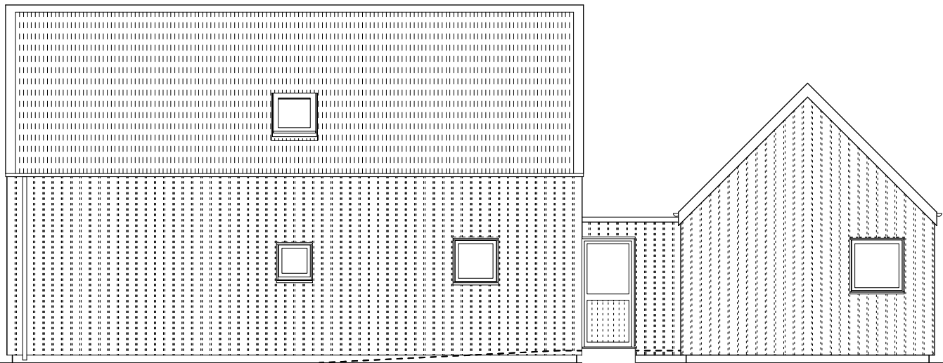
Elevation a
